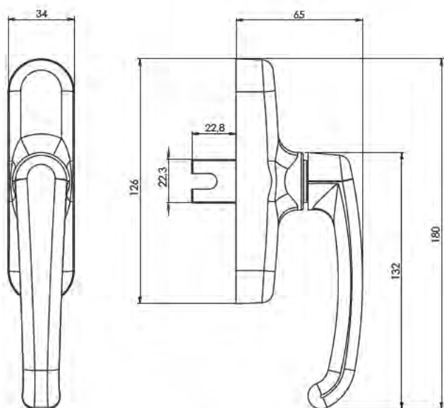
Вариант А Ручка стандартная
