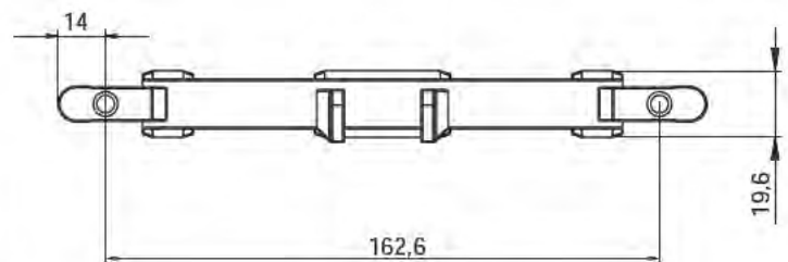
Вариант В под ручку с блокиратором
