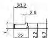
Подкладка ножниц люкс
