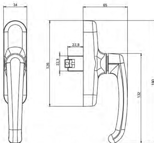
Вариант В Ручка с блокиратором
